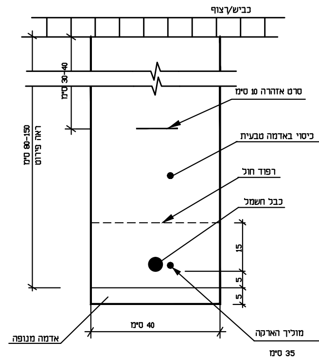
חתך טיפוסי צנור בחפירה
