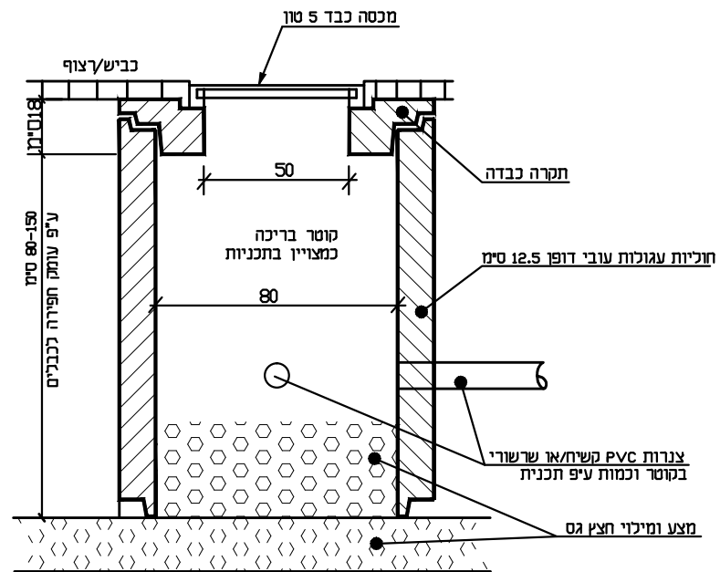
פרט בריכה מעבר
